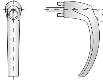
Fenstergriff für Falzgetriebe (rosettenlos)
