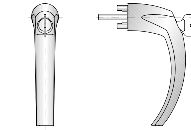
Fenstergriff für Falzgetriebe (rosettenlos)
